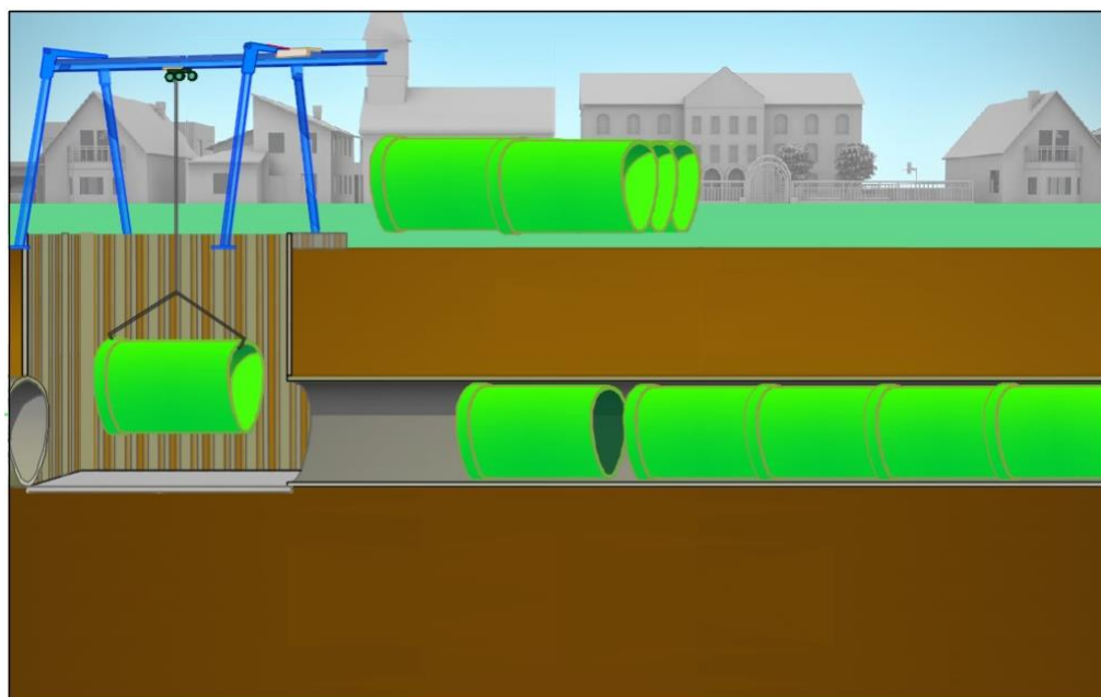
Abbildung 5: Kurzrohrverfahren mit Baugrube, Einfahrverfahren
