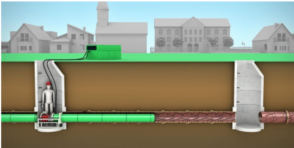
Abbildung 4: Kurzrohrverfahren (ohne) Baugrube, Einschubverfahren
